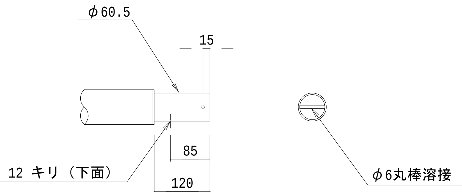
アダプター加工図
